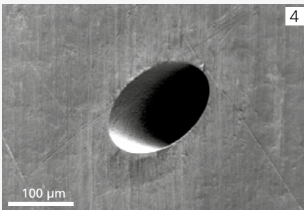
4 Bildausschnitt aus Abbildung 1: Elliptische Bohrung, 190 µm lang, 110 µm breit (REM-Aufnahme)
