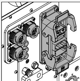
Industrietaugliche elektrische Anschlüsse (Ethernet, EtherCAT, Power, SPS, Laser) und LED-Status-Kontrollleuchten
