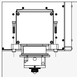
Montagebohrungen in der Nähe des Objektivs zur exakten Fixierung des Strahlaustritts (3-Punkt-Auflage)
