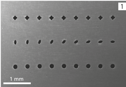
1 Flexible Geometrien in 300 µm Stahldicke (REM-Aufnahme, Austrittsseite)
